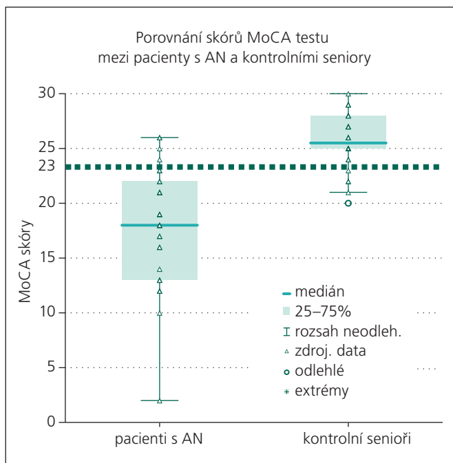
Graf 2. Porovnání skóre Montrealského kognitivního testu mezi pacienty s AN a kontrolními seniery podobného věku a vzdělání.
