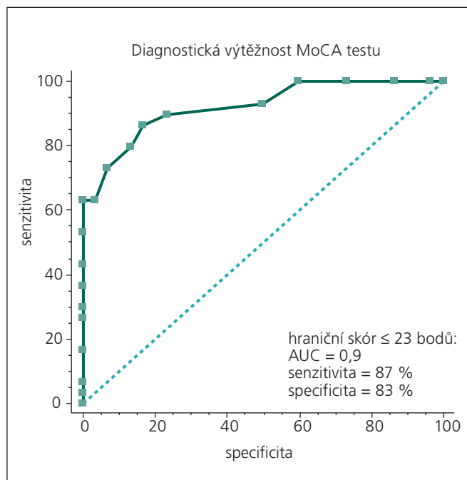
Graf 3. Křivka Receiver Operating Curve (ROC) porovnává senzitivitu proti specificku pro různé hraniční skóre Montrealského kognitivního testu.
