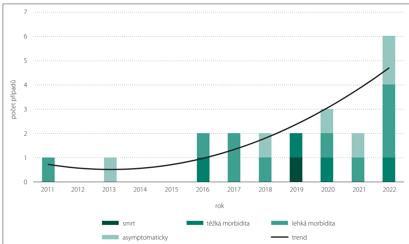
Obr. 1. Vývoj počtu případů a jejich závažnosti v čase. Černá linie představuje spojnicí trendu vyjádřenou jako polynomičnou křivku druhého stupně ( R^2 = 0,7311 ).
